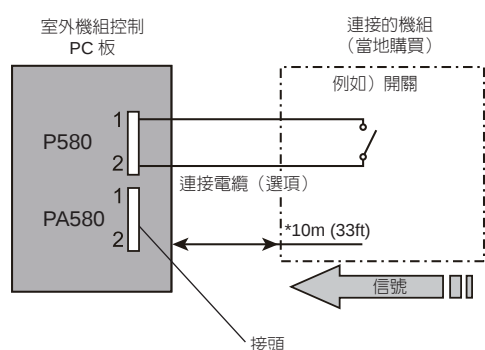
電路圖範例
