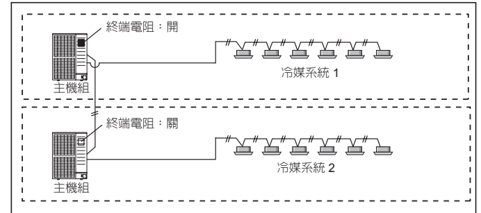
圖：終端電阻安裝
