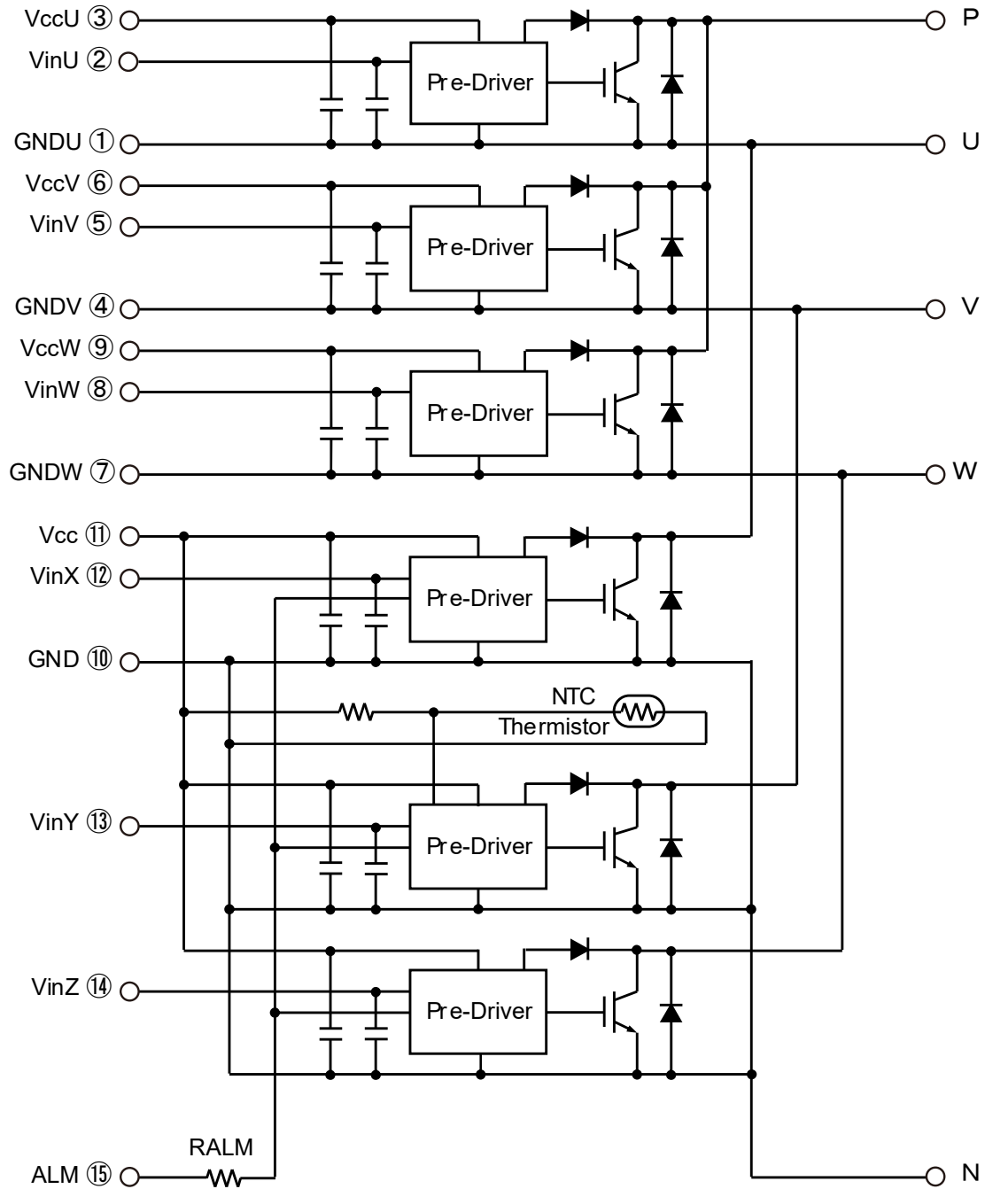
図 2. ブロック図
