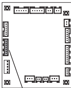
接收器單元端子 (CN13)
