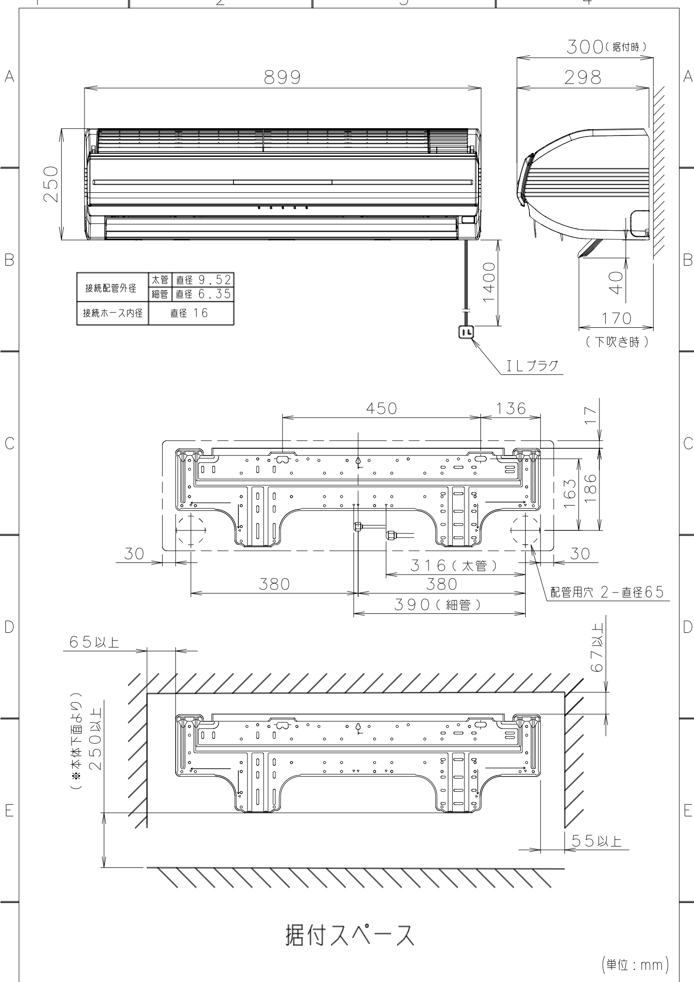
AS28PPZ-W 外形図及び据付板取付図(室内機)
